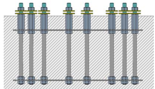
Verankerungssatz 2
